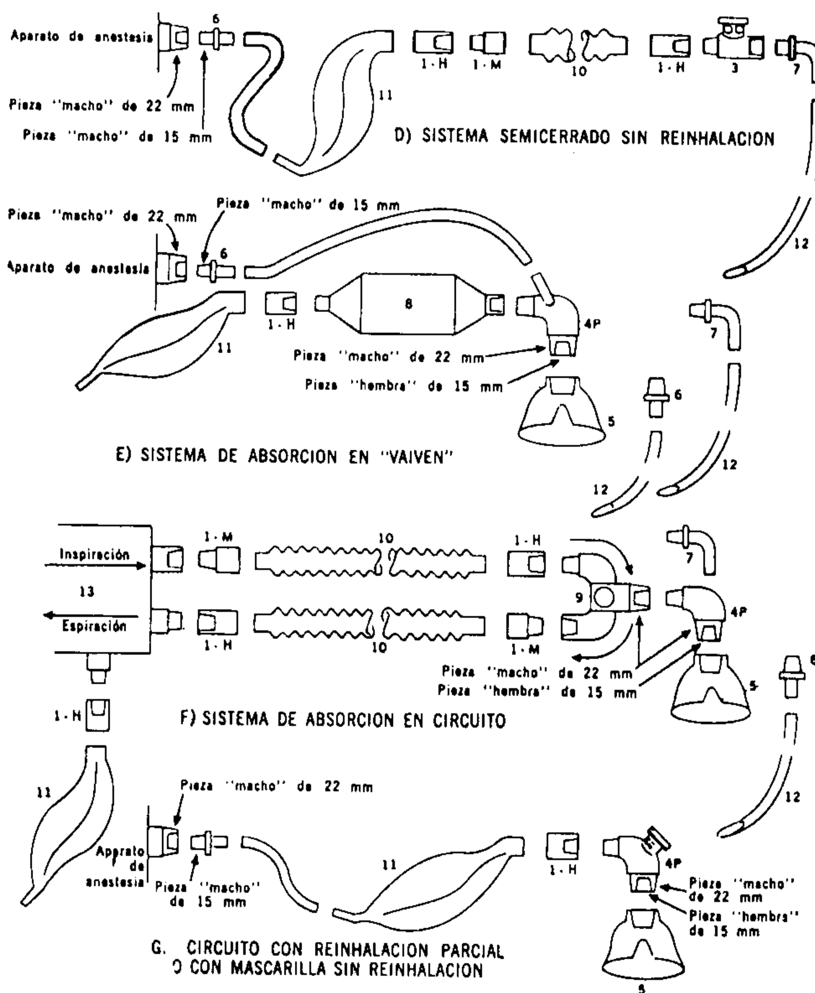
Fig. 1 Esquema padrão com relação aos equipamentos do aparelho de anestesia para uso em pediatria. No sistema pediátrico, a sucessão das partes e "macho - fêmea" na direção do fluxo gasoso.
