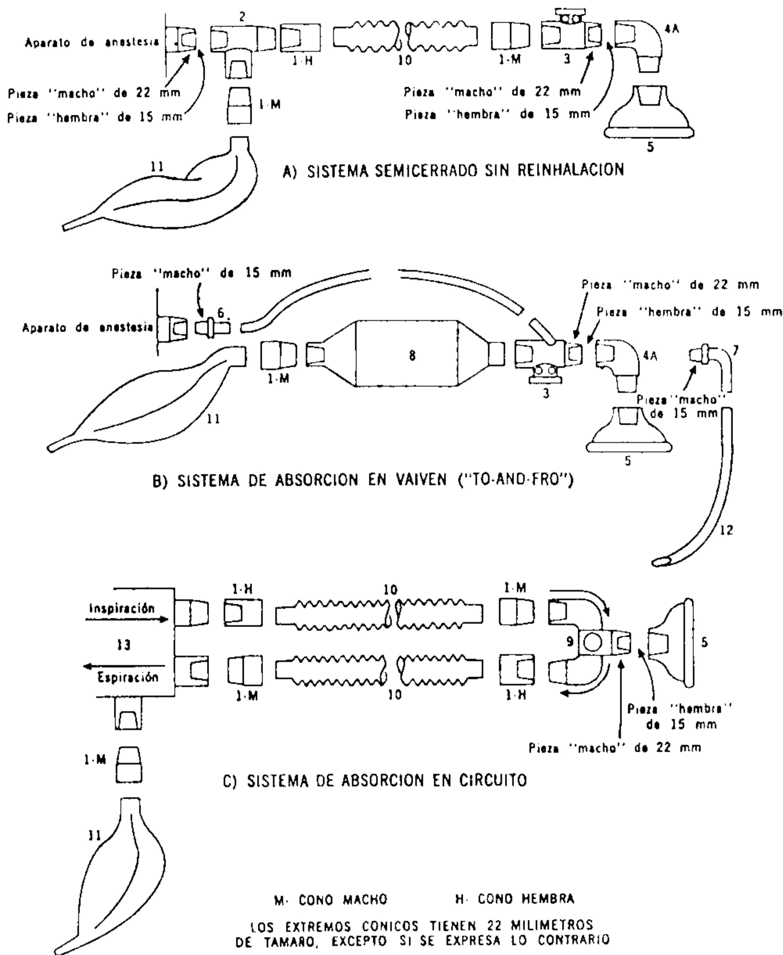
Fig. 2 Esquemas padrões, recomendados para sistemas de ventilação e acessórios do aparelho de anestesia para adultos.
